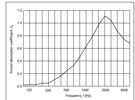
Ljudtest Figur 4: Montering: De 11 panelerna ligger platt på betonggolvet i ekotestrummet. Stängd ram runt kanten.
