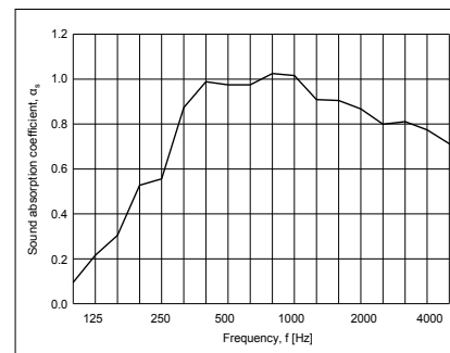
Ljudtest Figur 3: Montering: 45 mm luftavstånd bakom panelen. Stängd ram runt kanten.
